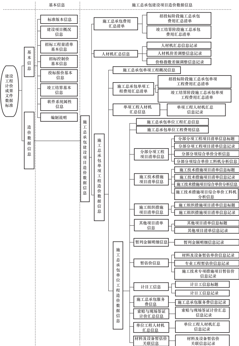
图 3-1 建设项目施工总承包数据信息结构图
